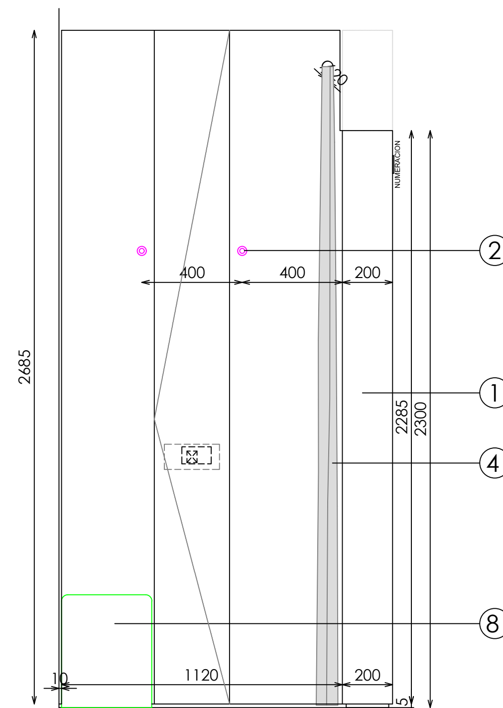
ALZADO LATERAL CUELGA (B-B)
