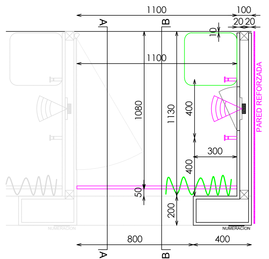
PLANTA
