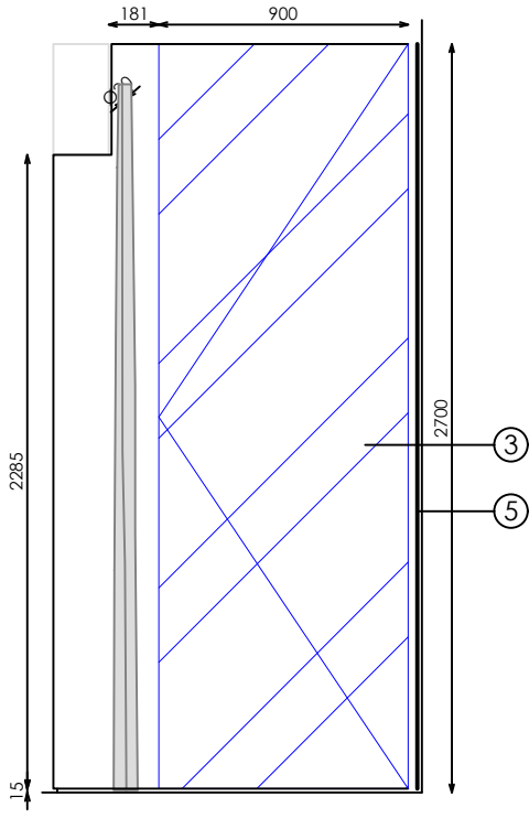
ALZADO LATERAL ESPEJO (A-A)
