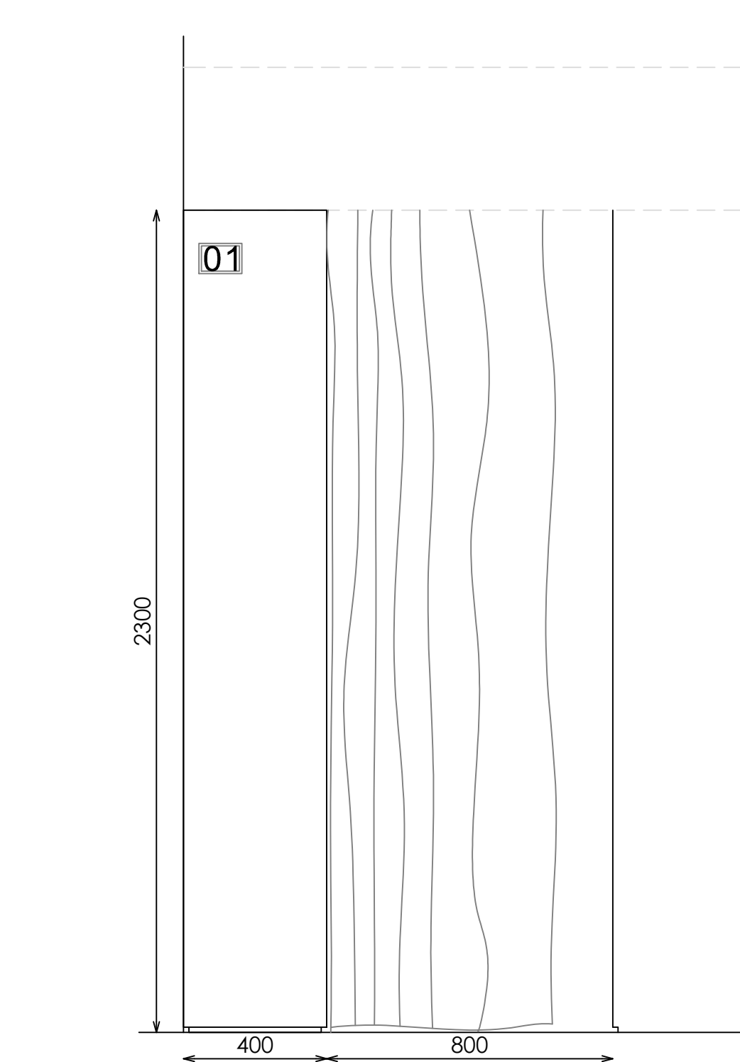
ALZADO
