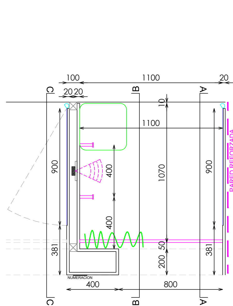
PLANTA
