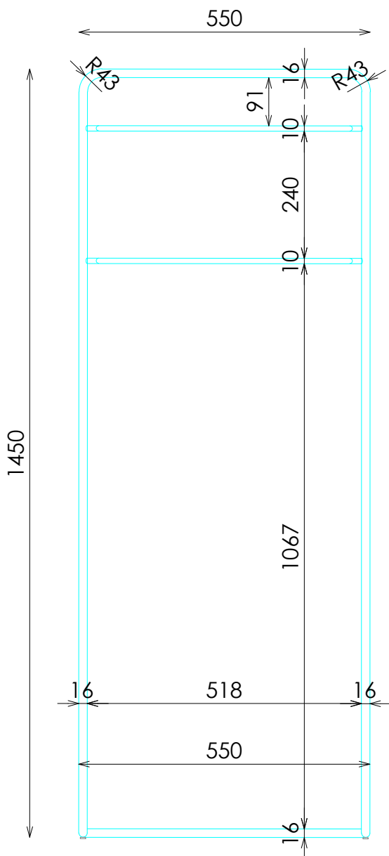
ALZADO FRONTAL
