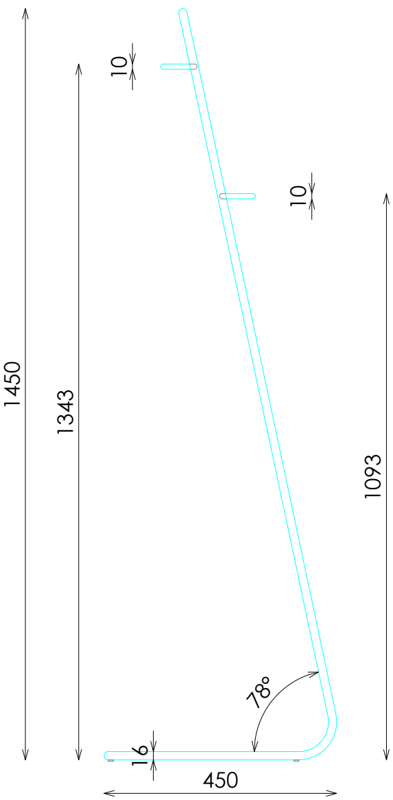
ALZADO LATERAL
