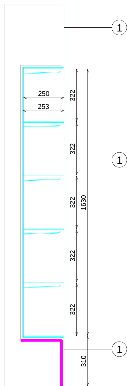
SECCION CALCETINES
