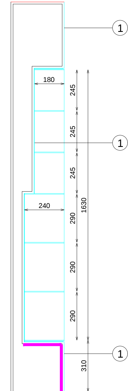
SECCION CAMISETAS
