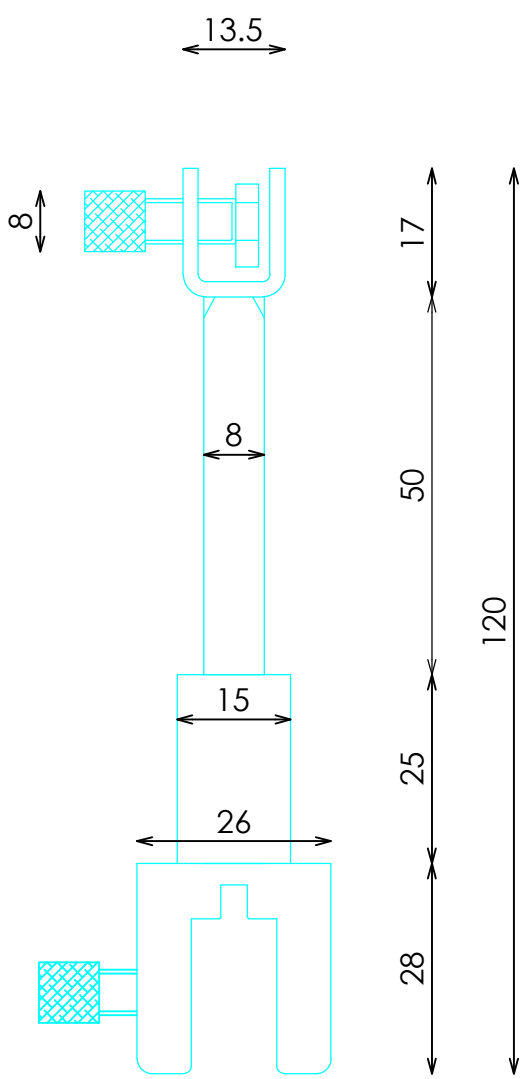
PERFIL
