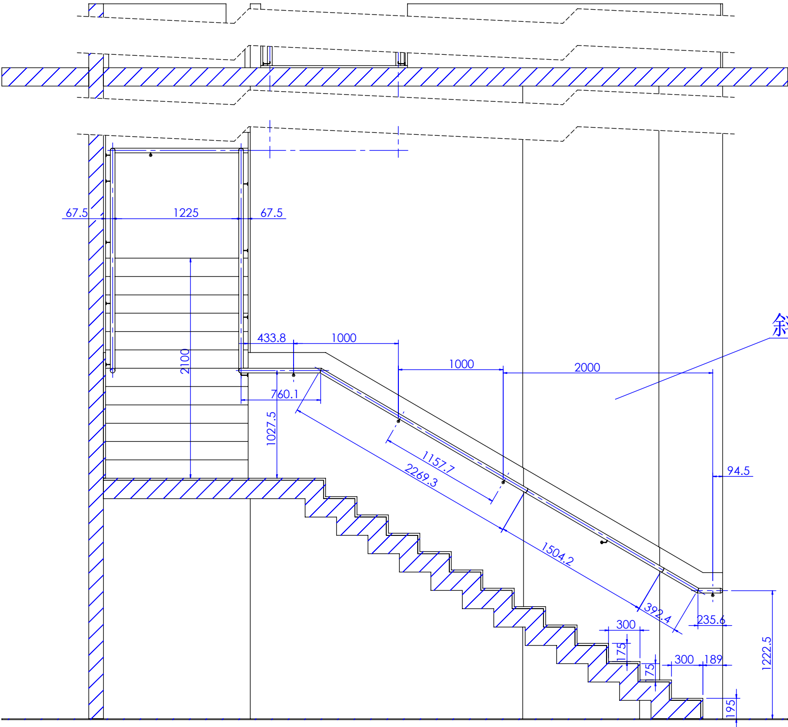
剖面 AN-AN
