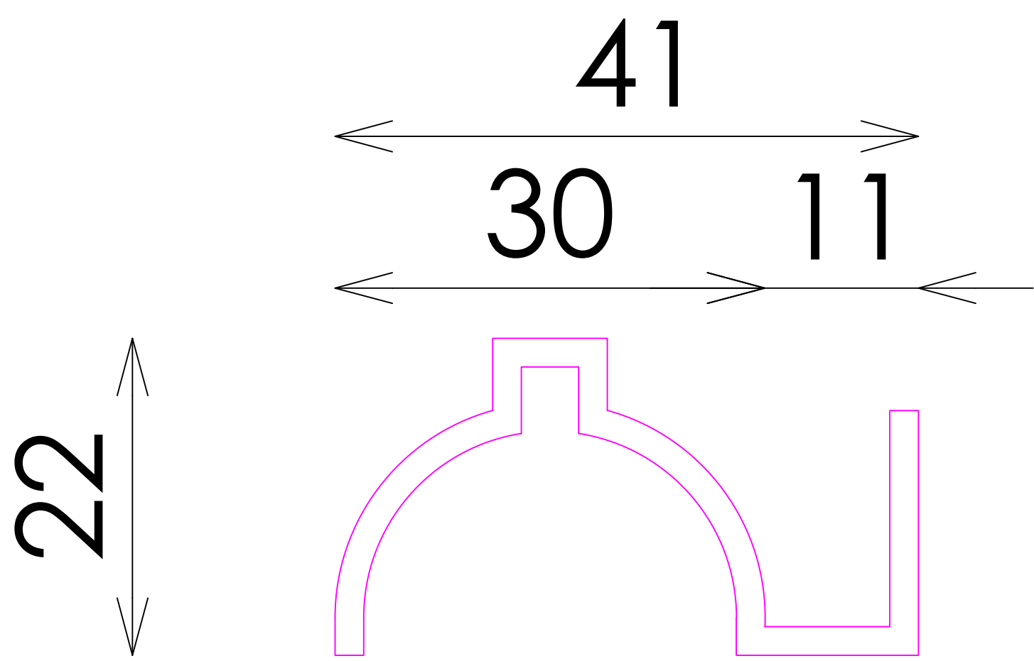
PERFIL
