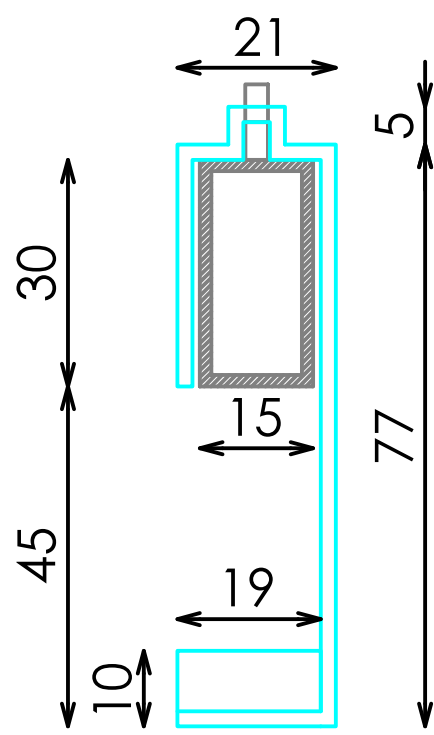
SECCIÓN
