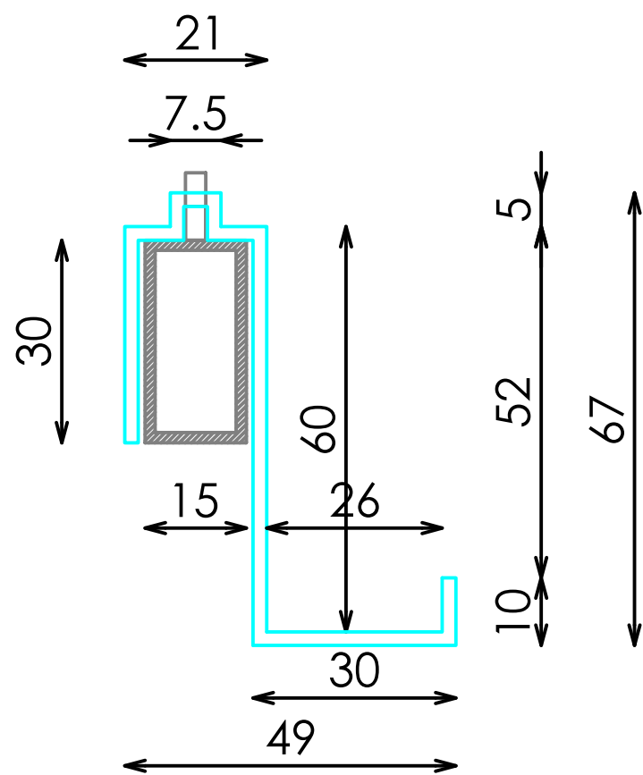
SECCIÓN
