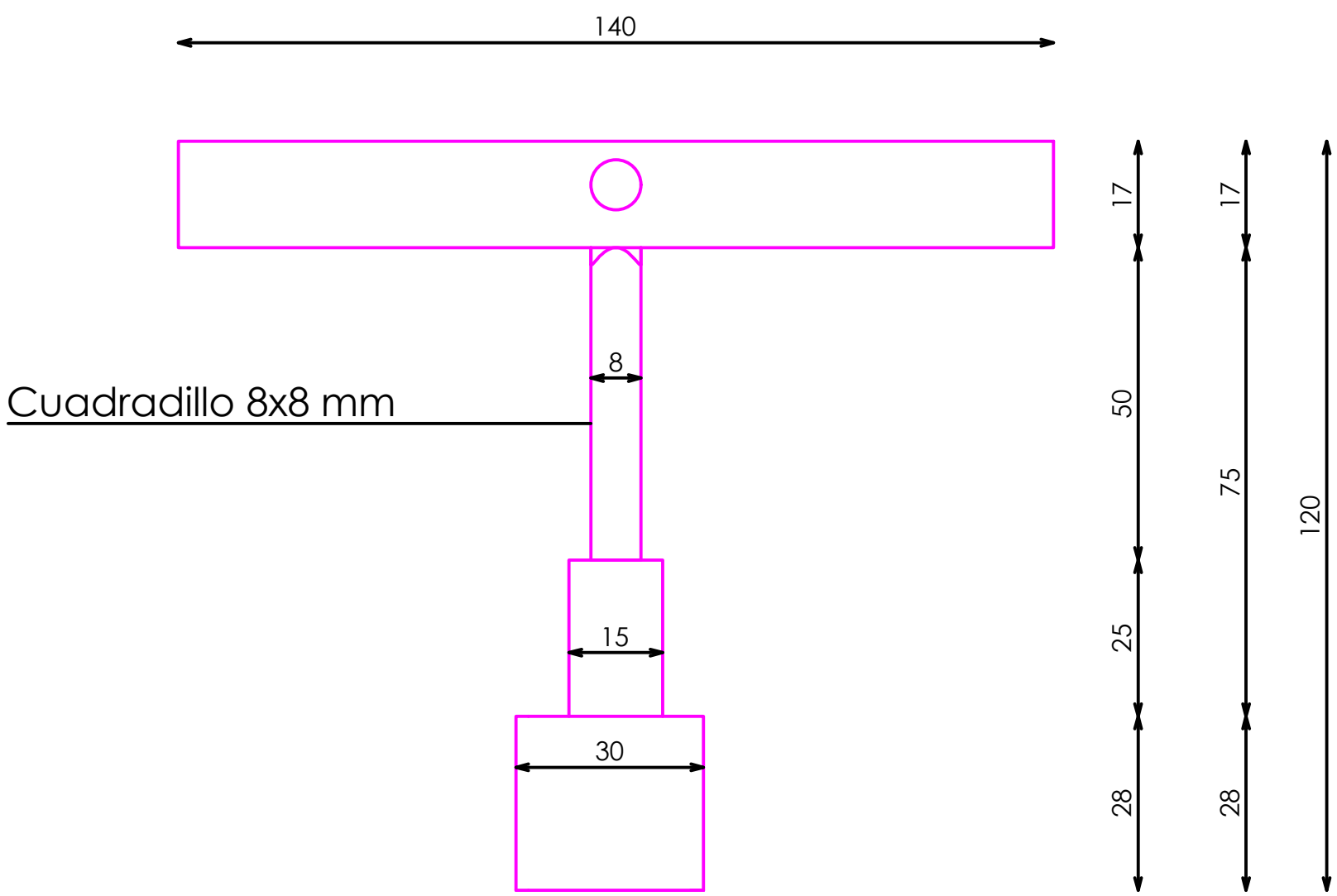
ALZADO
