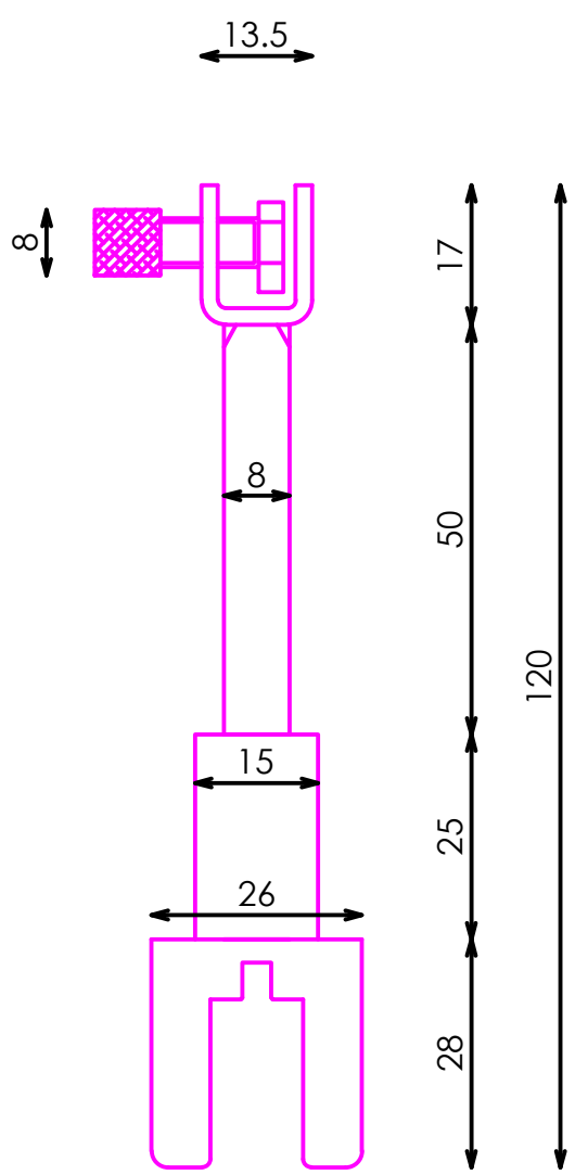
PERFIL
