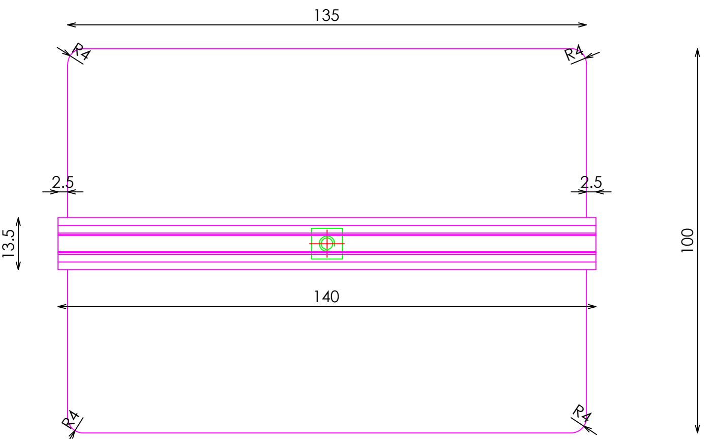
PLANTA
