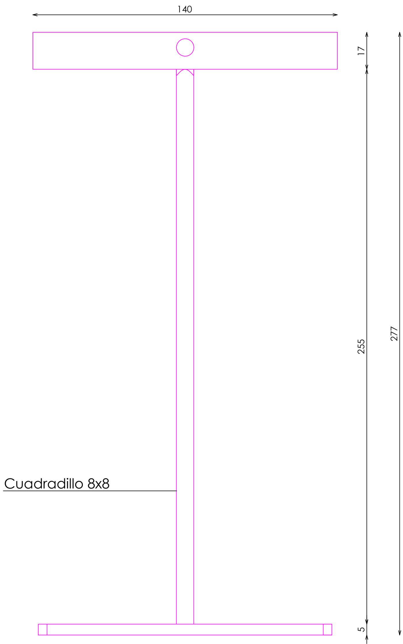
ALZADO
