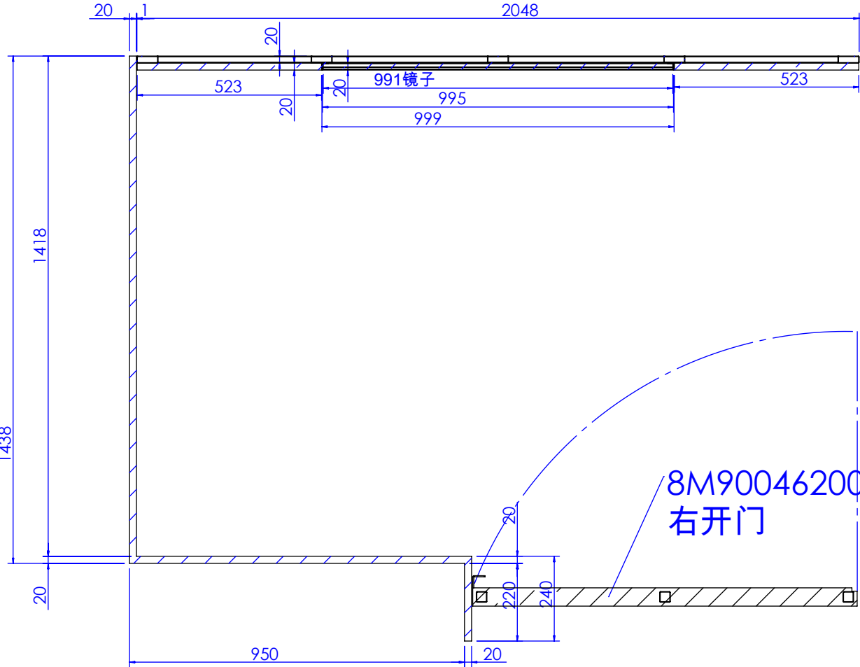
剖面 AG-AG 比例 1 : 15
