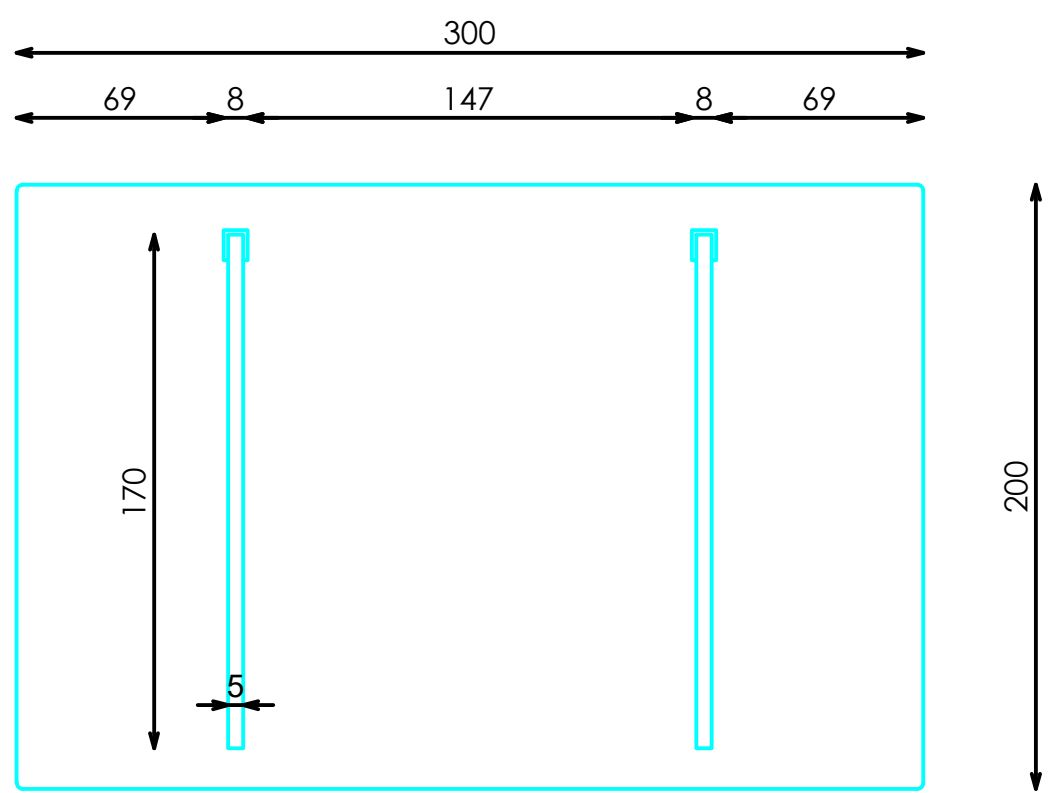
PLANTA
