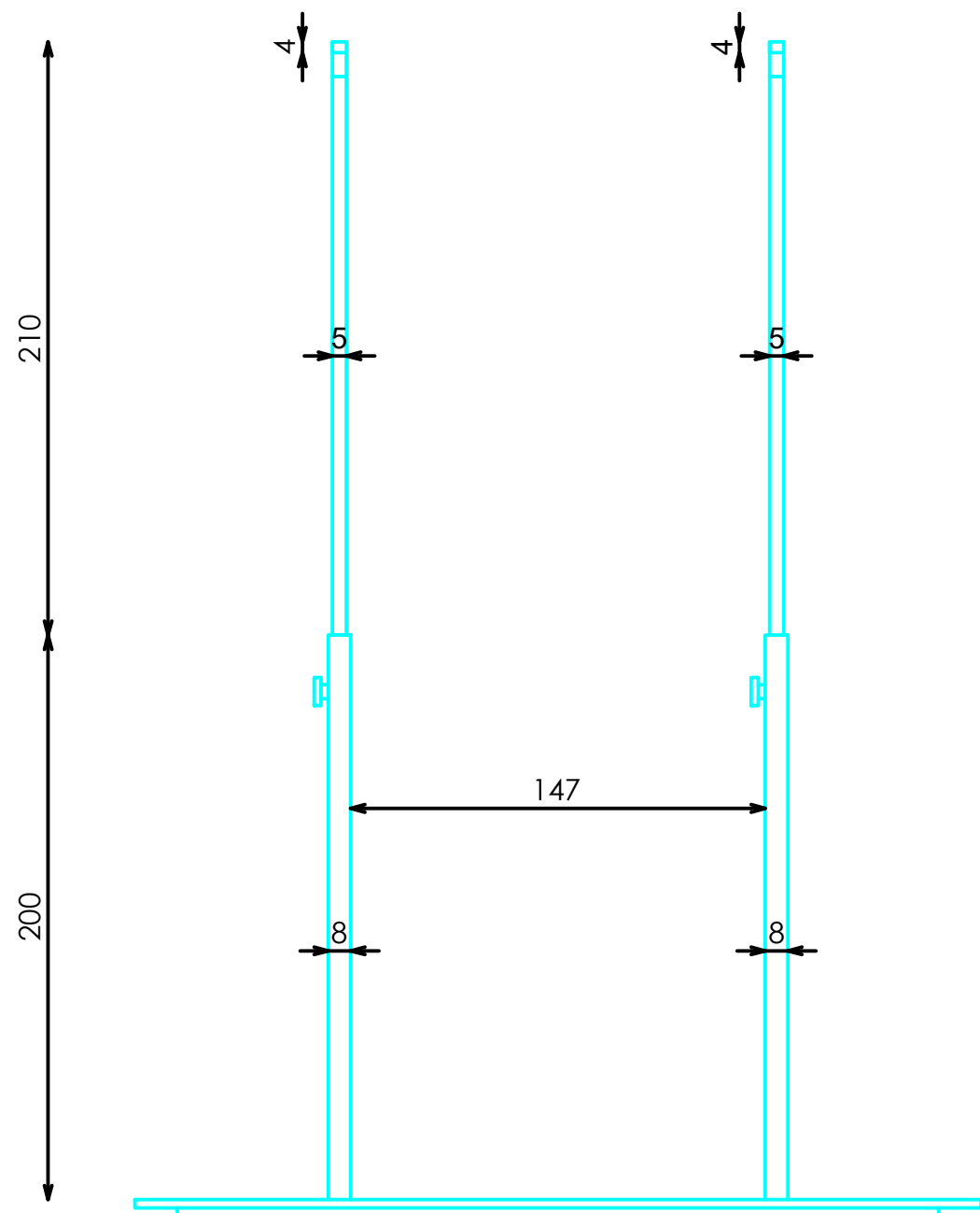
ALZADO
