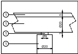
DETALLE B
