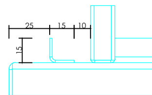
DETALLE E
