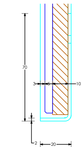
DETALLE A
