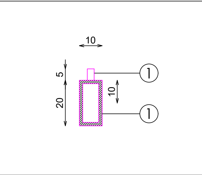
DETALLE A
