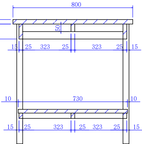
剖面 A-A
