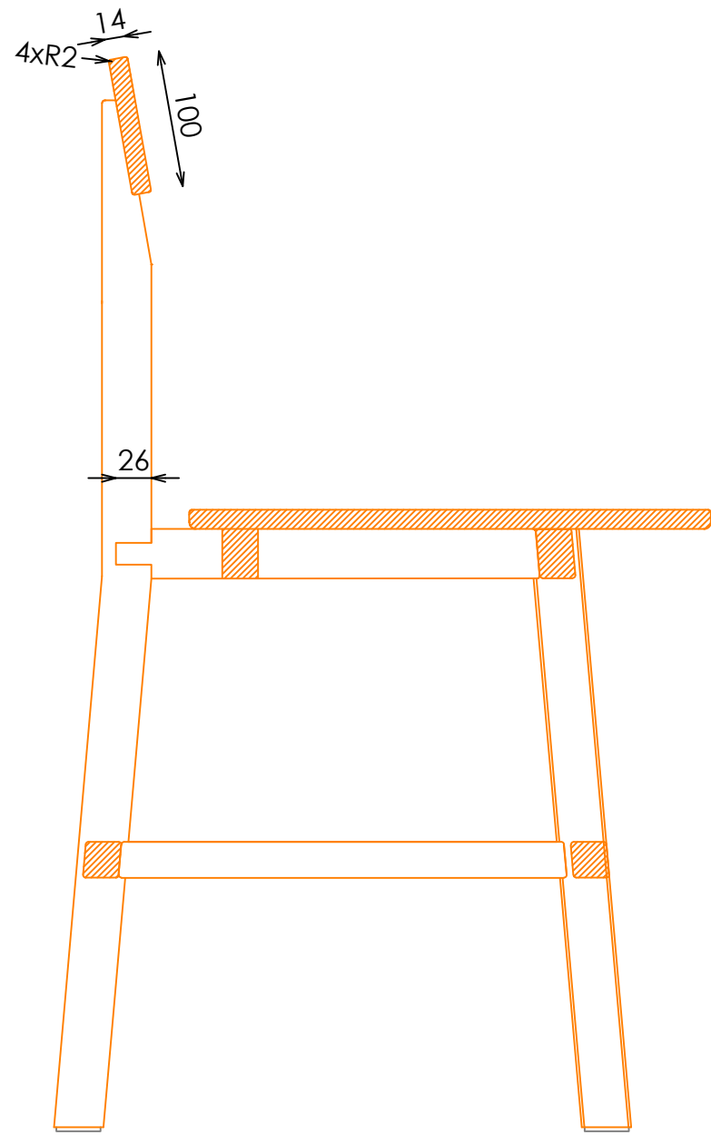
SECCION C-C
