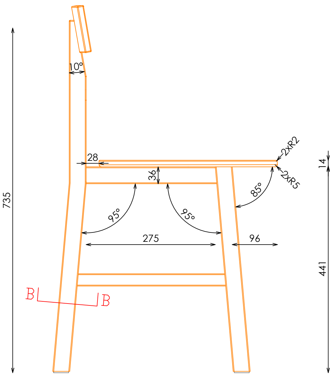
ALZADO LATERAL
