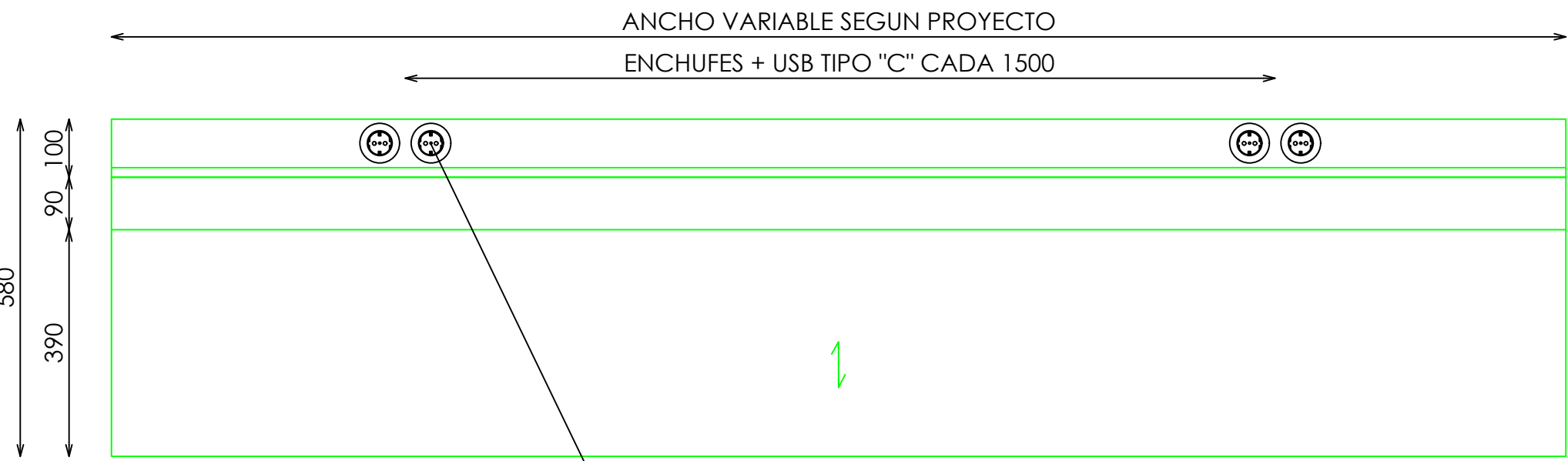
PLANTA
