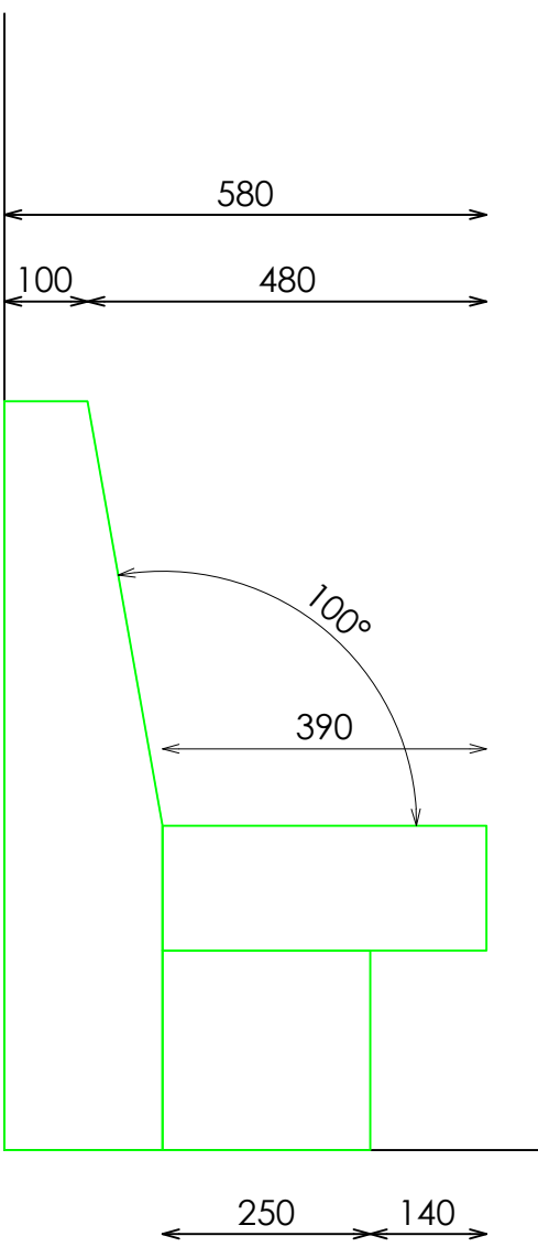
PERFIL
