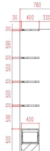
剖面 B-B
