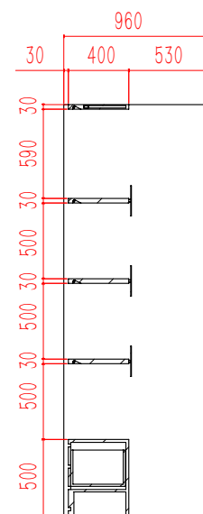
剖面 E-E
