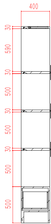
剖面 F-F
