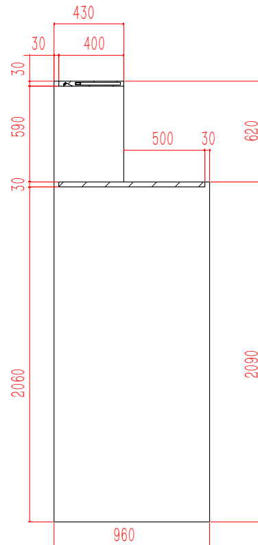
剖面 H-H
