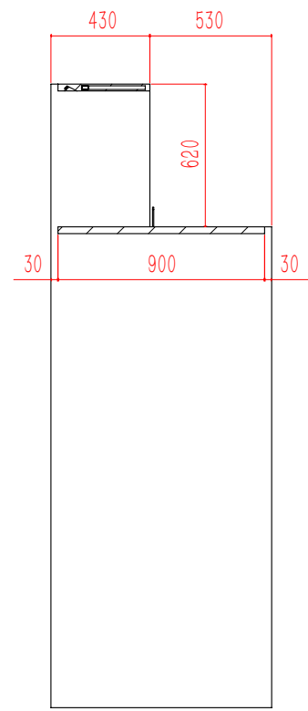
剖面 G-G
