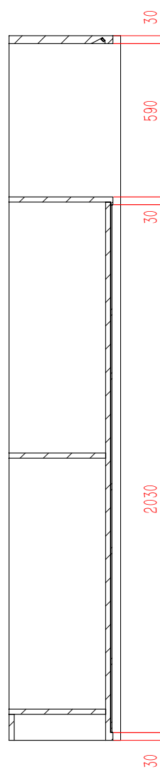
剖面 E-E
