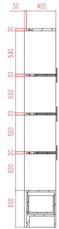
剖面 B-B
