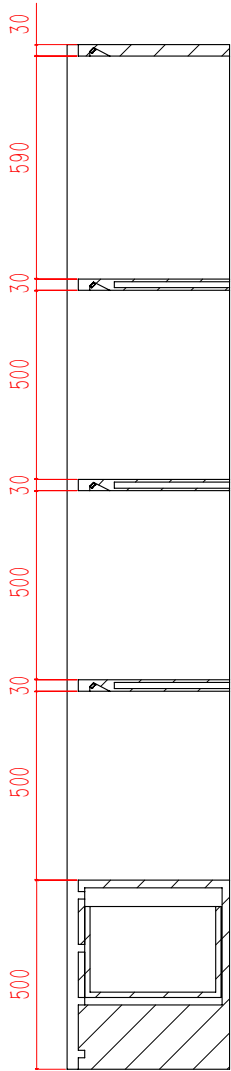
剖面 F-F
