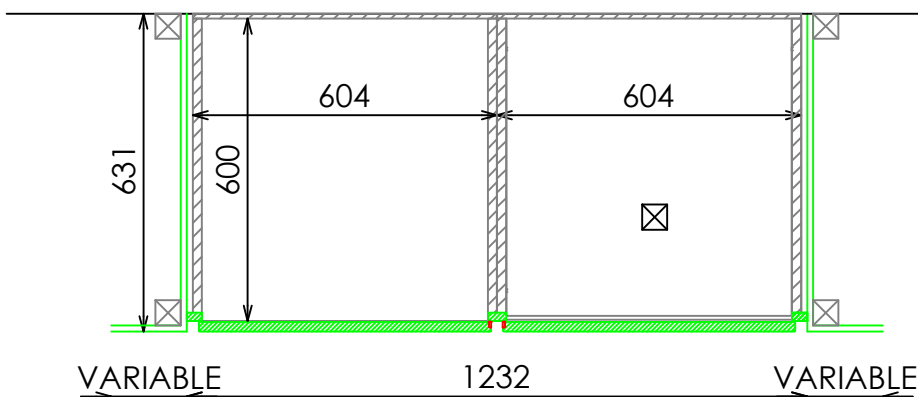
PLANTA
