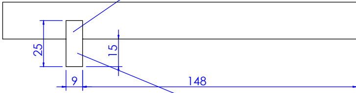
局部视图 AG 比例 1 : 2
