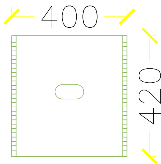
ALZADO 2 ELEVATION 2
