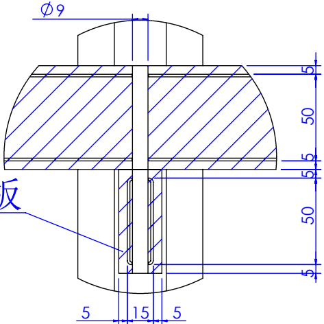
局部视图 AN 比例 1:2
