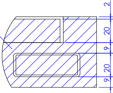
局部视图 AN 比例 1:2
