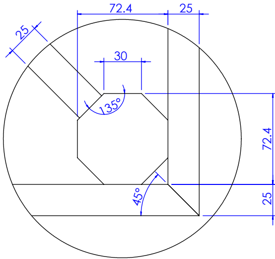
局部视图 AO 比例 1:3
