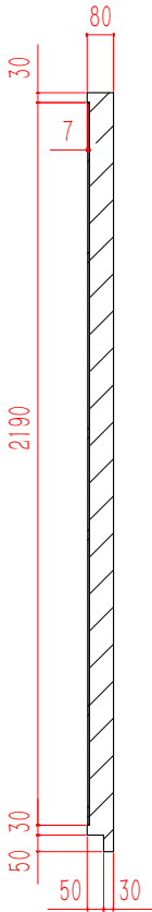
剖面 E-E
