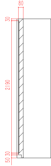
剖面 C-C
