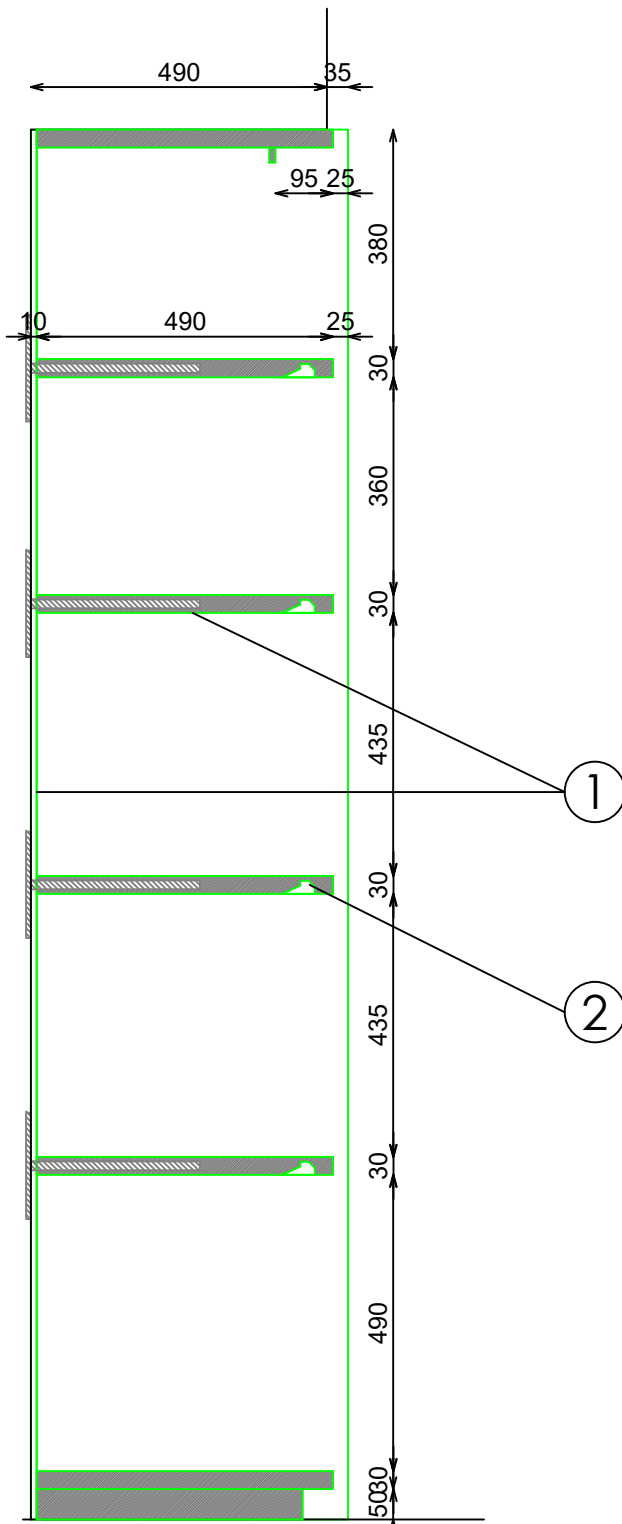
SECCION
