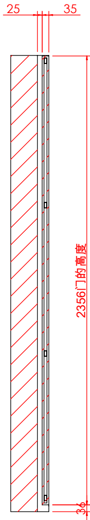
剖面 AG-AG
