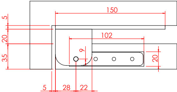
局部视图 AH
