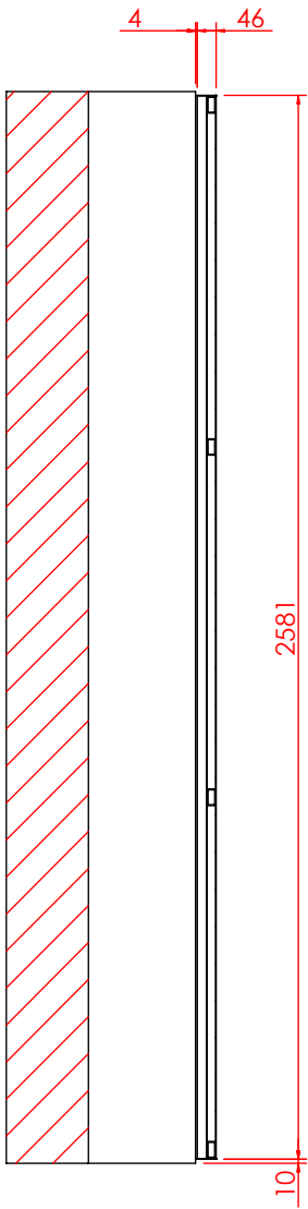
剖面 AM-AM
