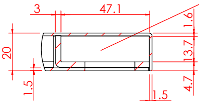
局部视图 AK 比例 1:2
