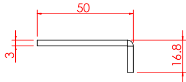
局部视图 AL 比例 1 : 2
