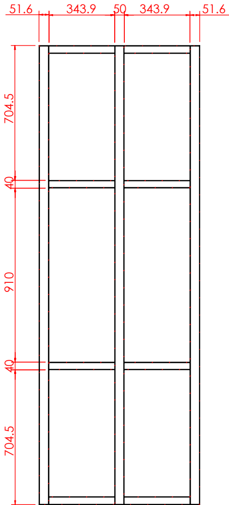
剖面 AJ-AJ
