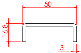
局部视图 AM 比例 1 : 2
