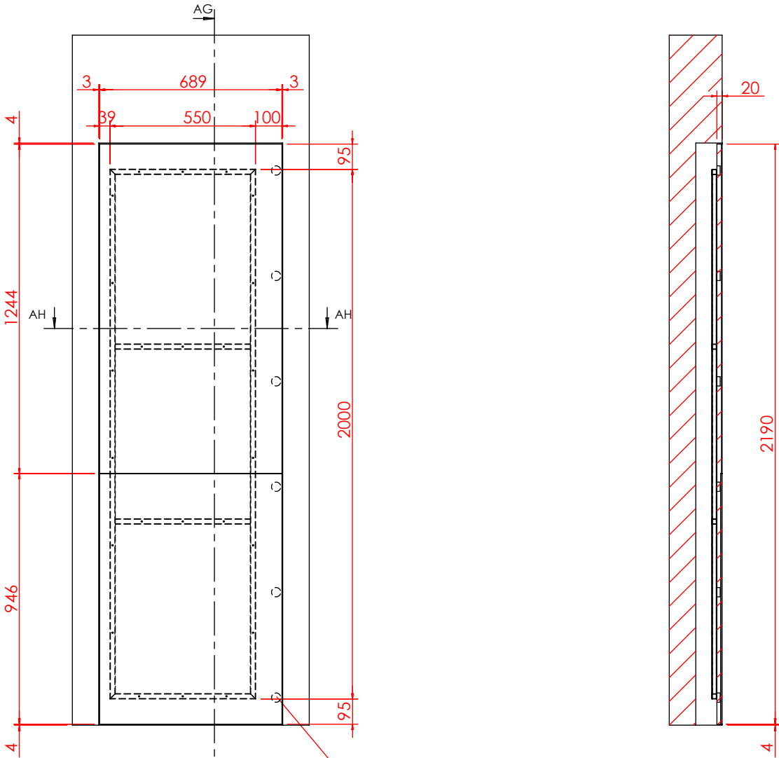
剖面 AG-AG
