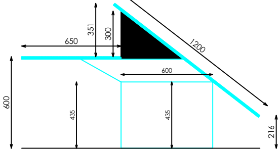
SECCIÓN A-A
