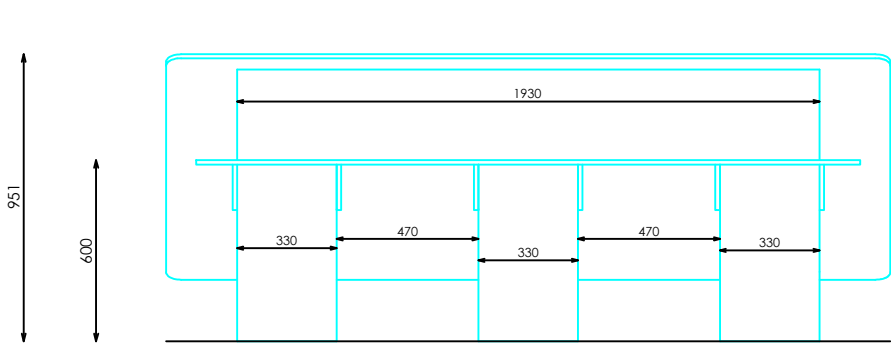
ALZADO POSTERIOR
