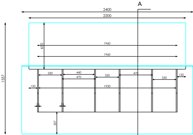
ALZADO FRONTAL
