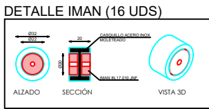
SECCIÓN A-A
