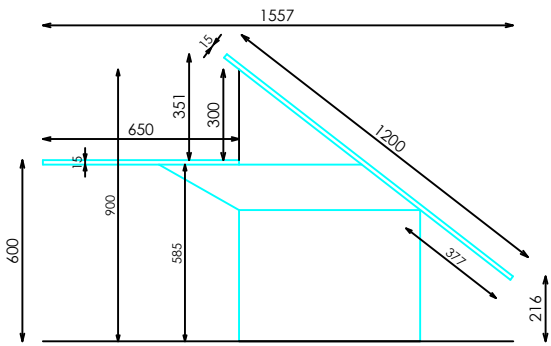
ALZADO LATERAL
