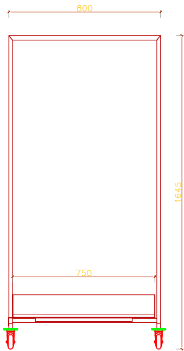
ALZADO FRONTAL
