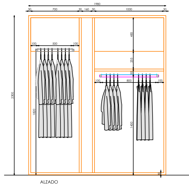
ALZADO
