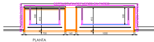
PLANTA
