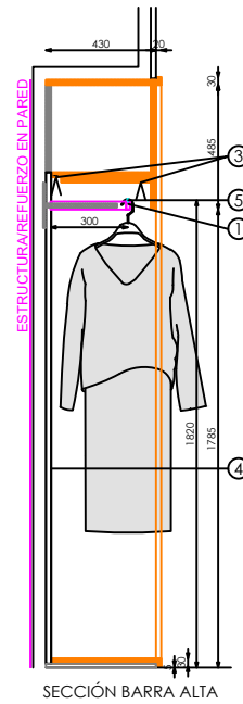
SECCIÓN BARRA ALTA
