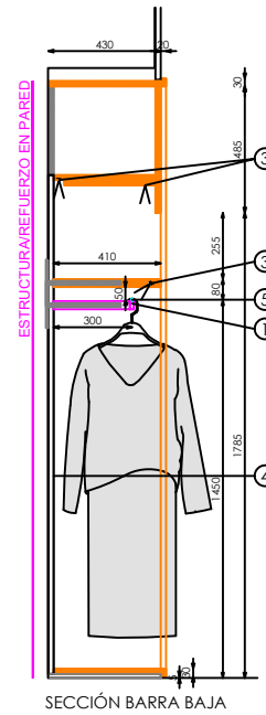
SECCIÓN BARRA BAJA
