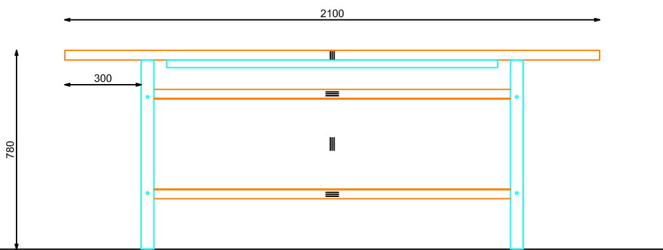
ALZADO FRONTAL
