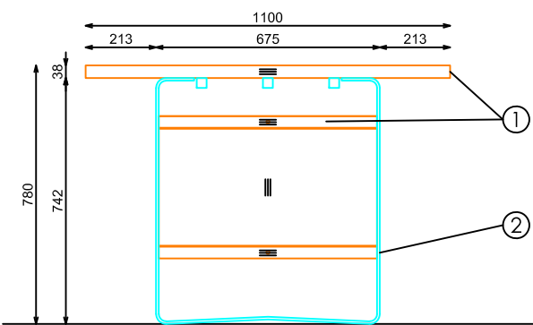
ALZADO LATERAL
