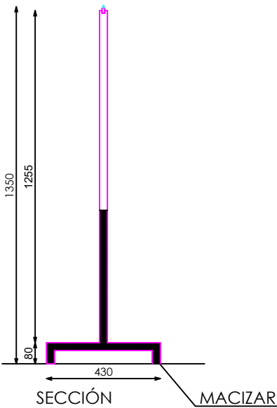
SECCIÓN
