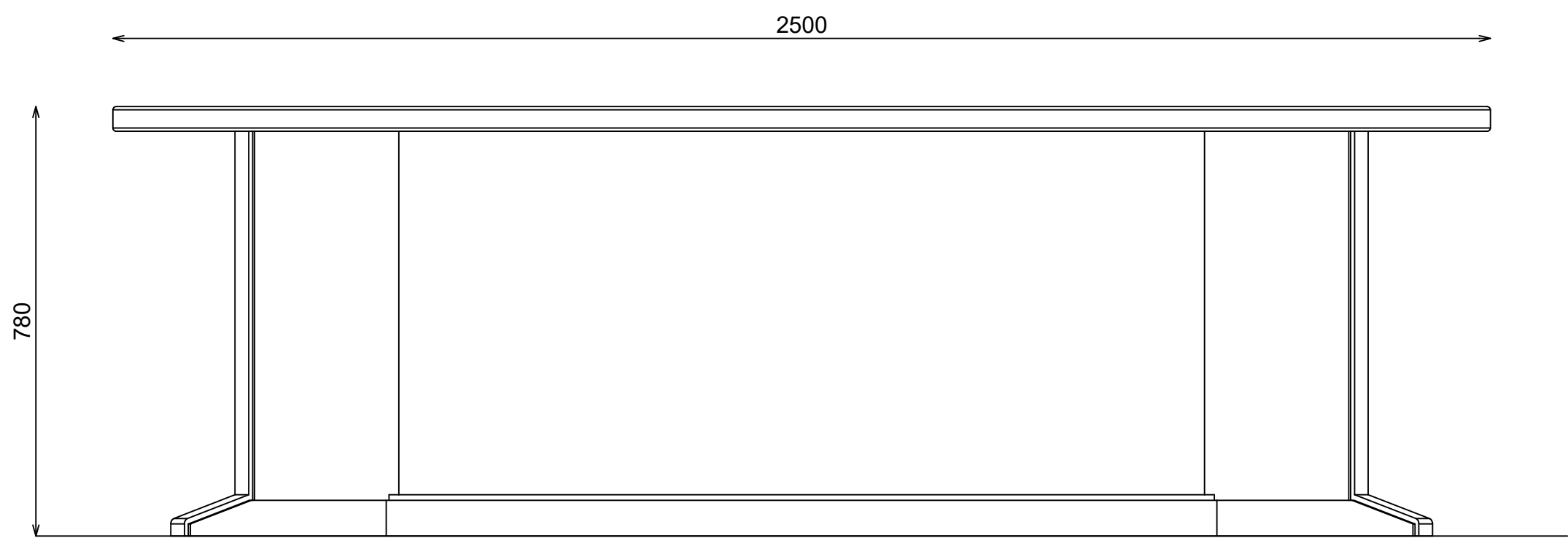
ALZADO
