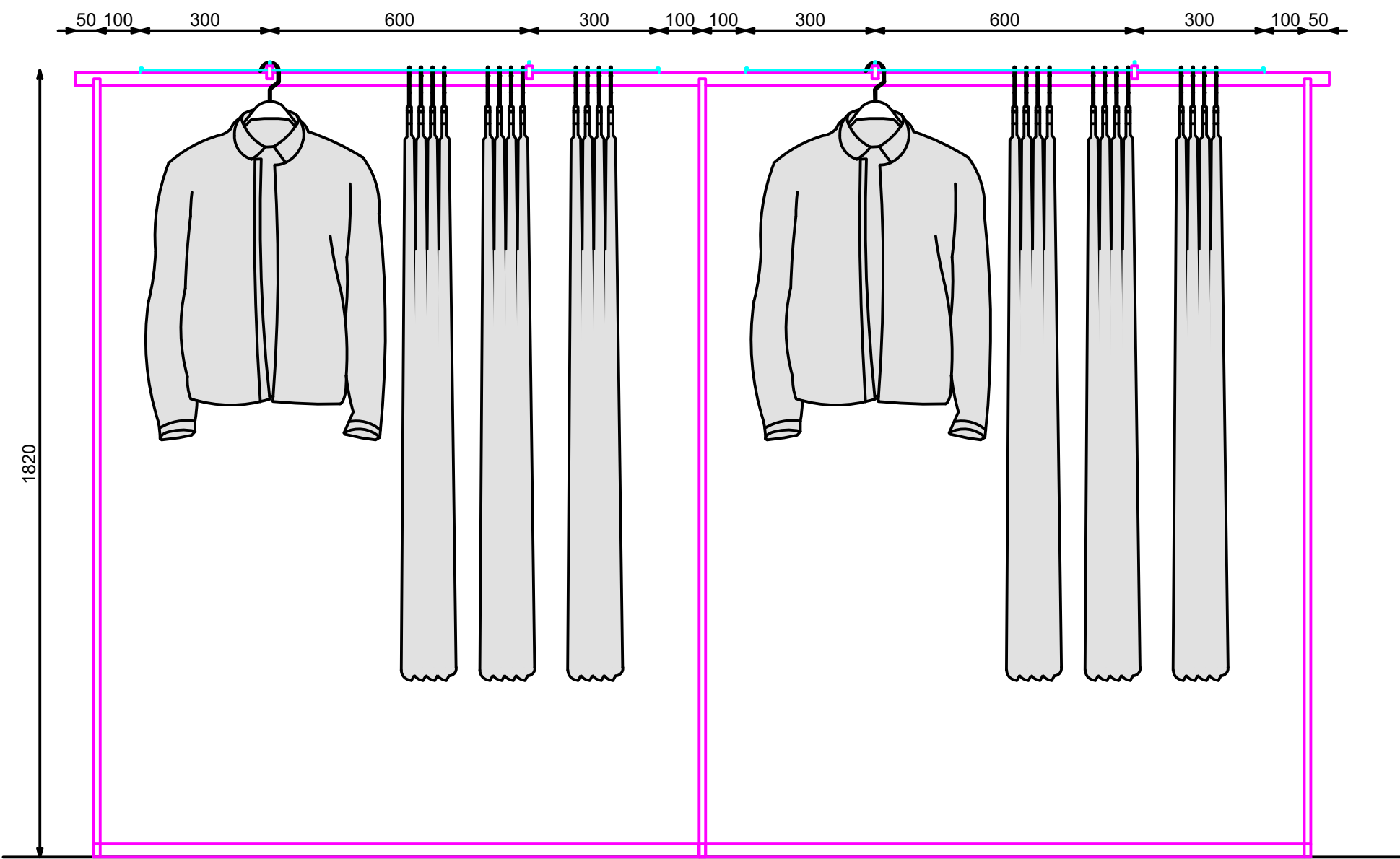
ALZADO
