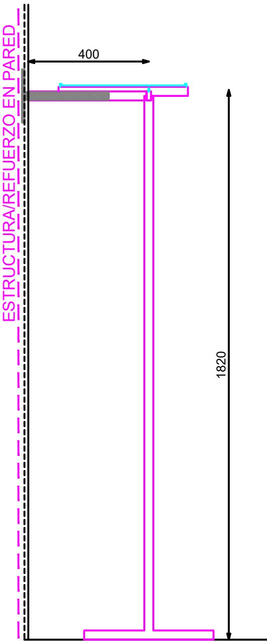
SECCION
