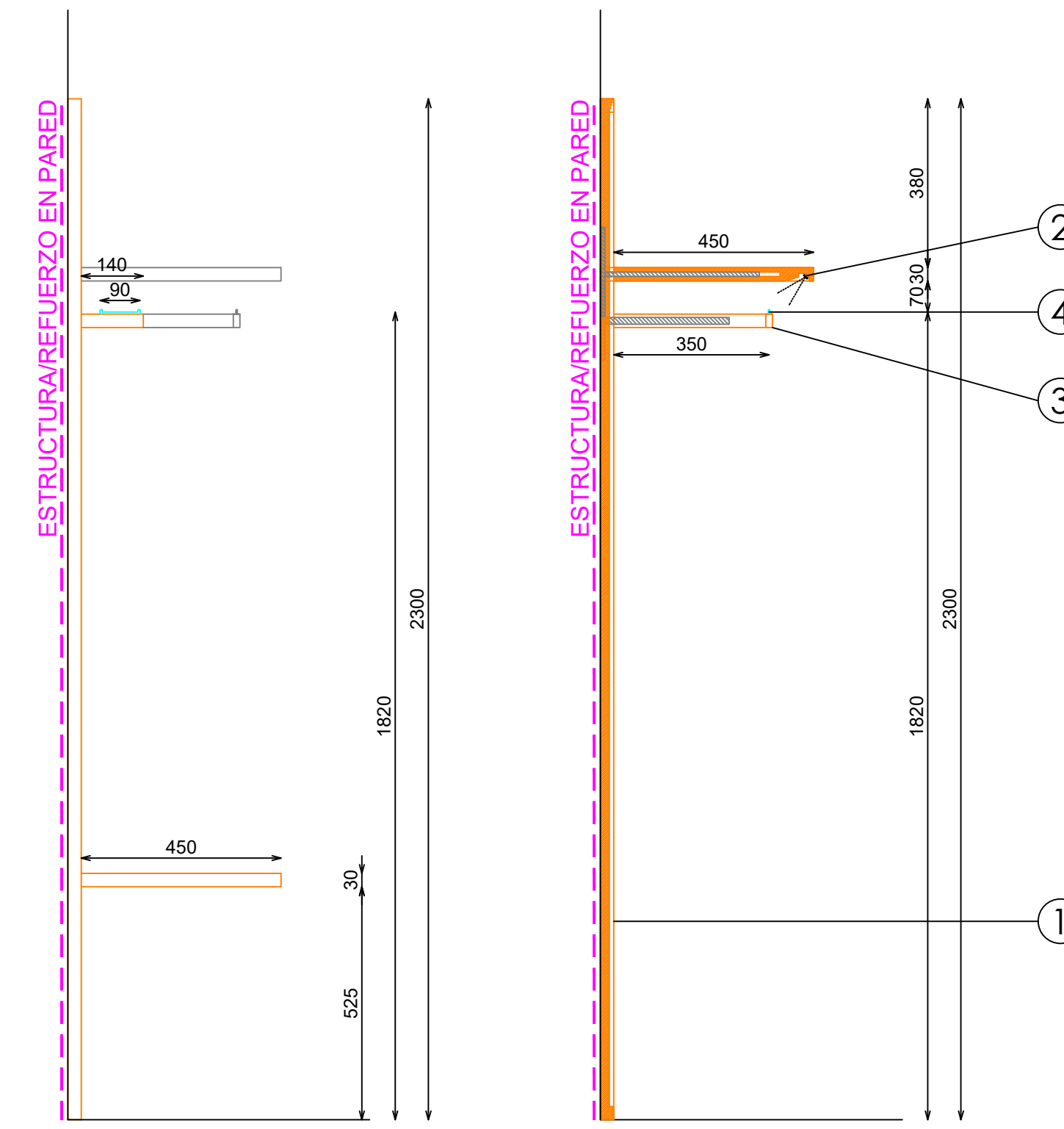
ALZADO LATERAL
