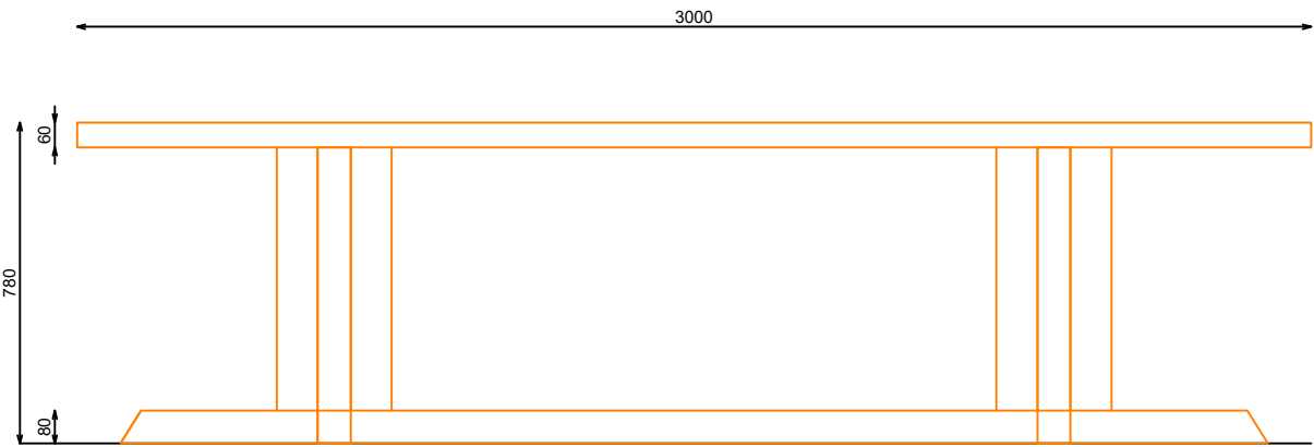
ALZADO FRONTAL
