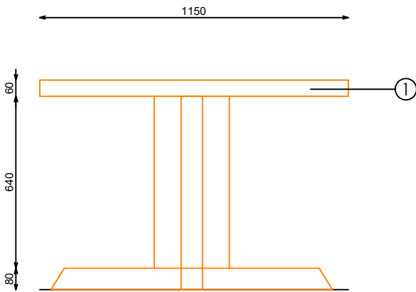
ALZADO LATERAL
