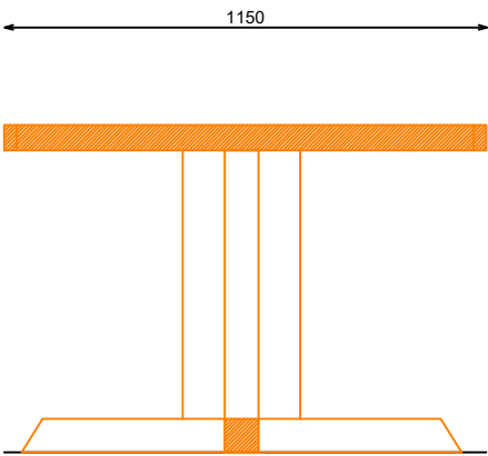
SECCION
