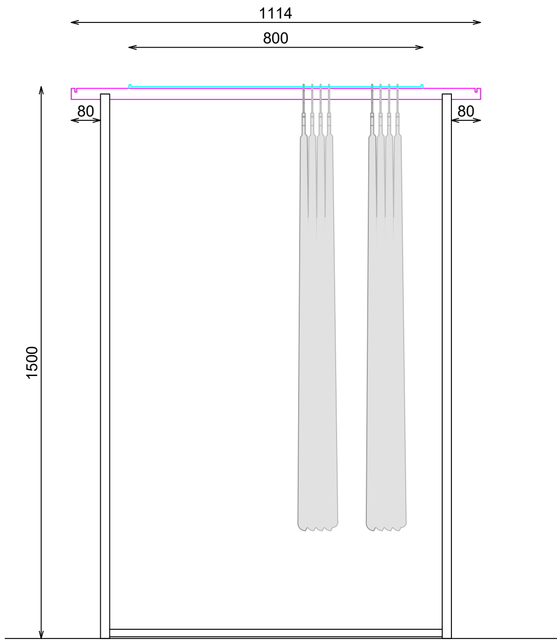
ALZADO
