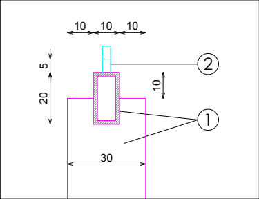
DETALLE A
