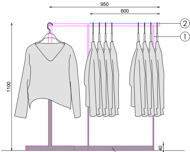
ALZADO LATERAL
