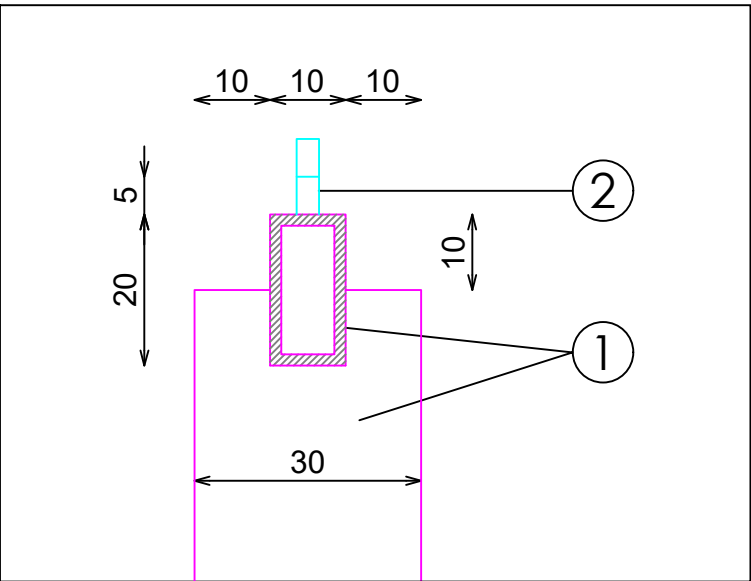
DETALLE B
