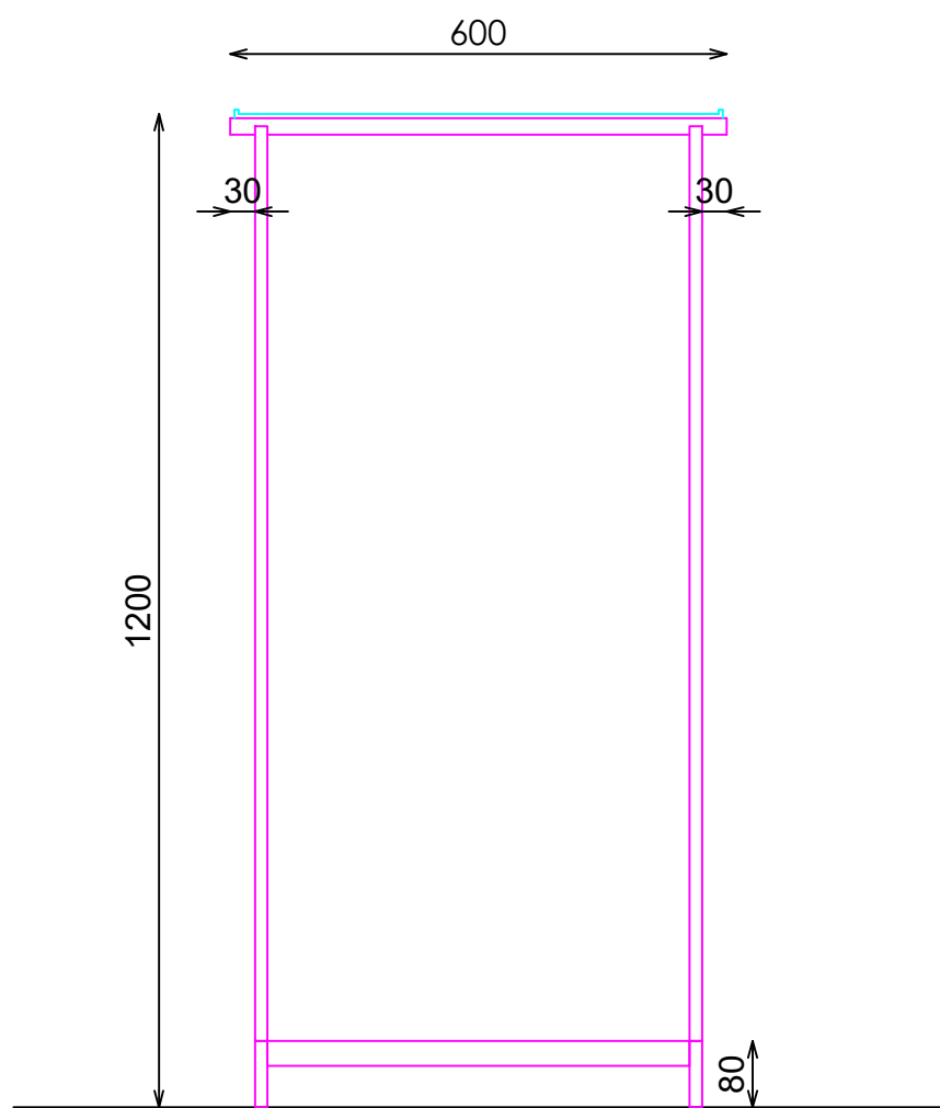
ALZADO
