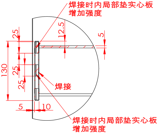
局部视图 D 比例 1 : 4
