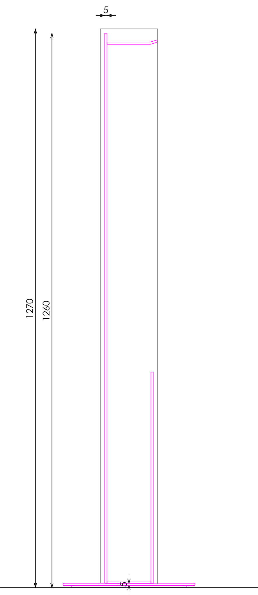
PERFIL SECCIONADO
