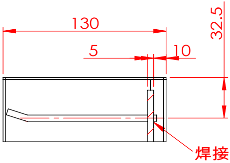
局部视图 C 比例 1 : 3
