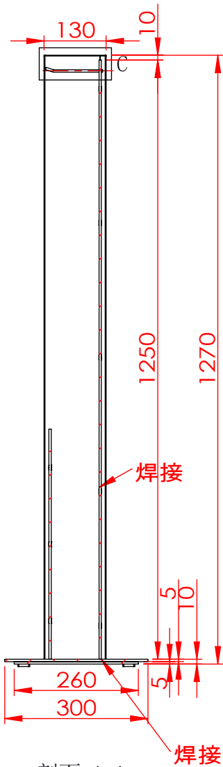
剖面 A-A
