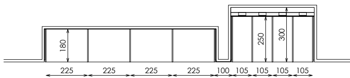
PLANTA A-A
