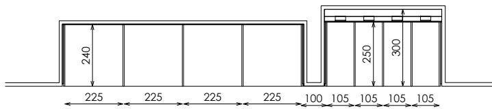
PLANTA B-B
