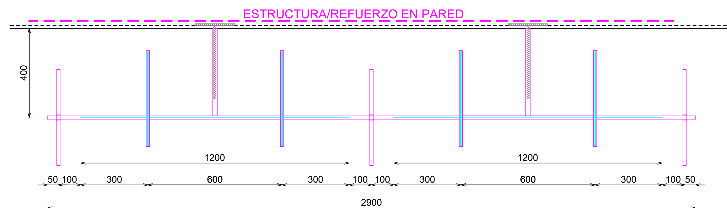
PLANTA
