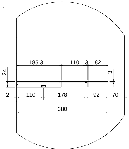
局部视图 AJ 比例 2 : 15
