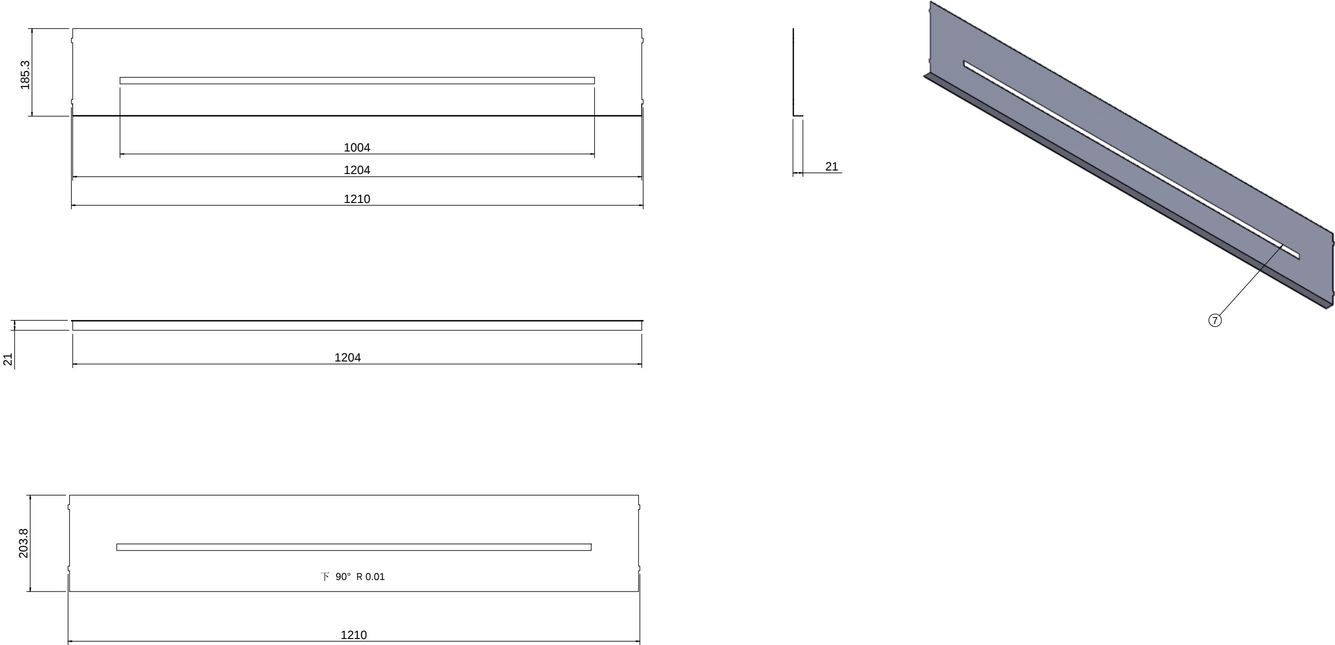
金属展开图
