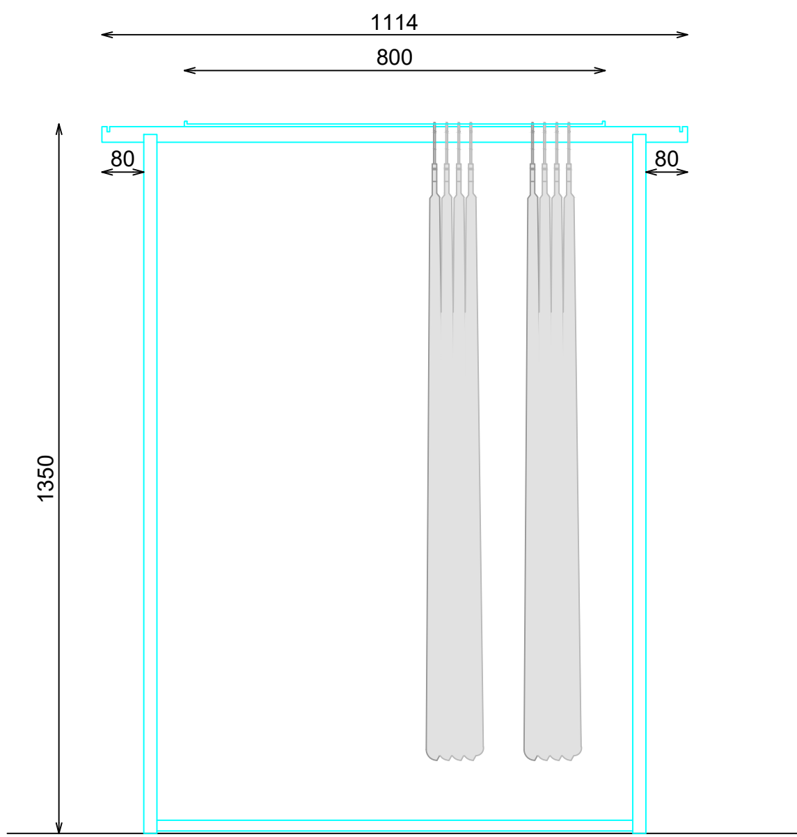
ALZADO
